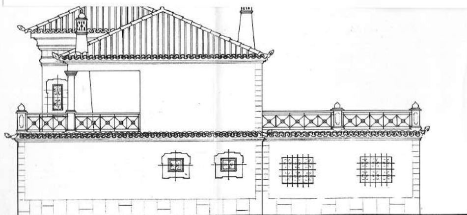
ALÇADO NASCENTE
