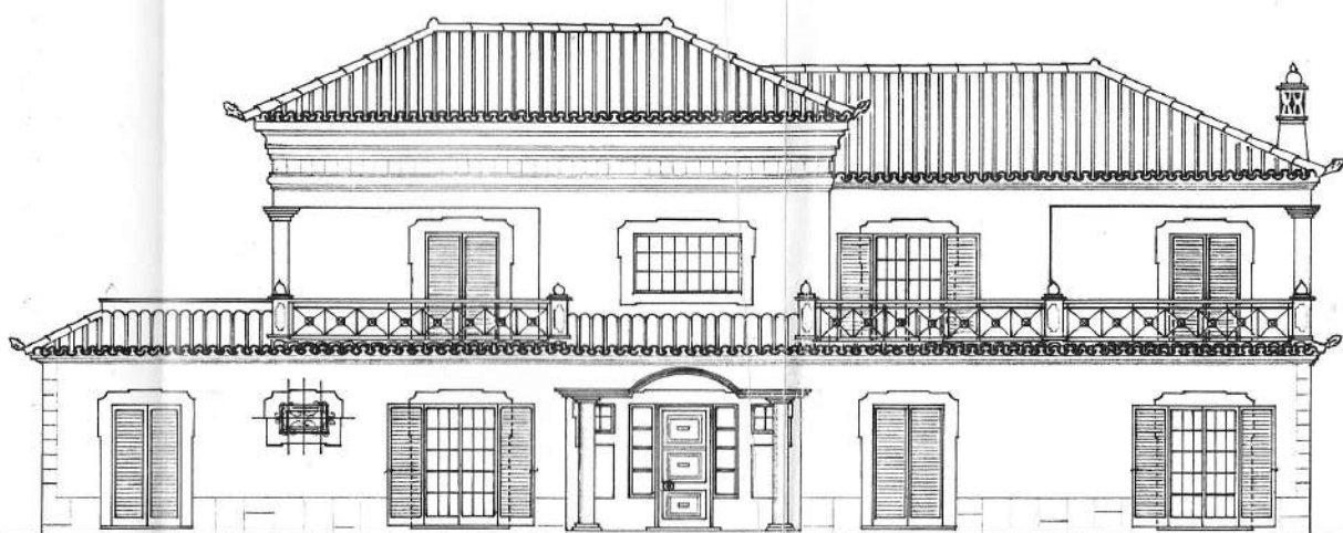
ALÇADO SUL
