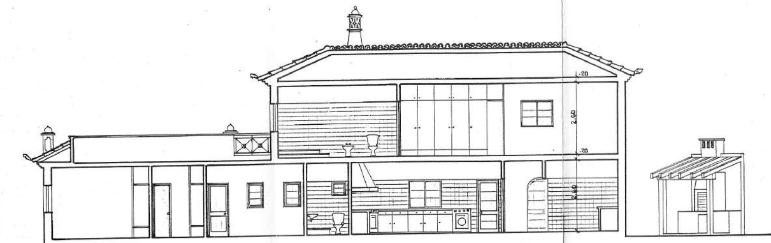
CORTE A-B
