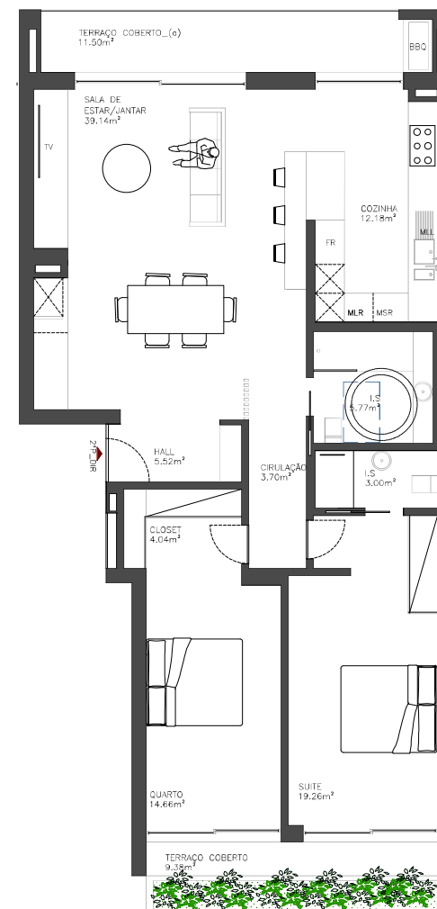
PLANTA LOTE 11 _ 2º direito_2º PISO
