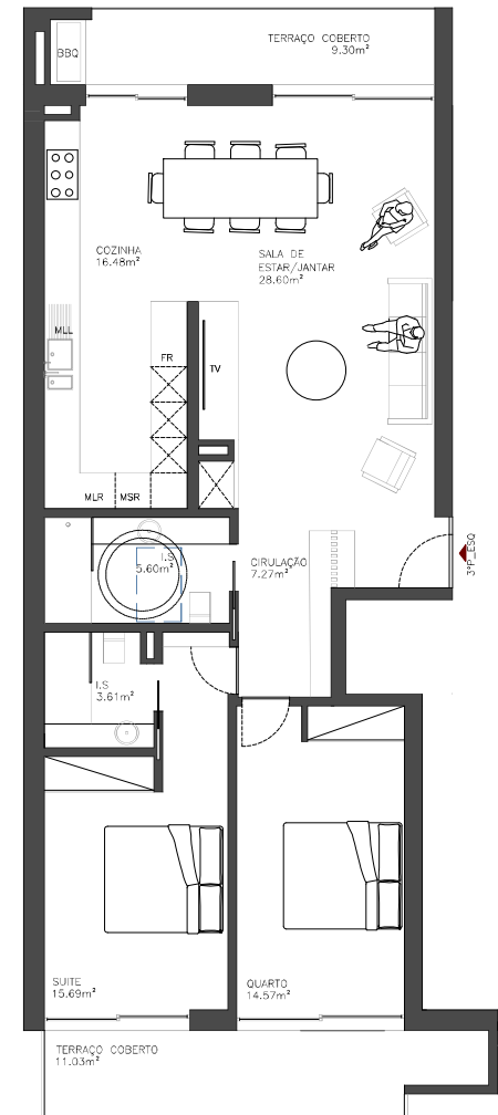
PLANTA LOTE 11_3º ESQUERDO_3º PISO
