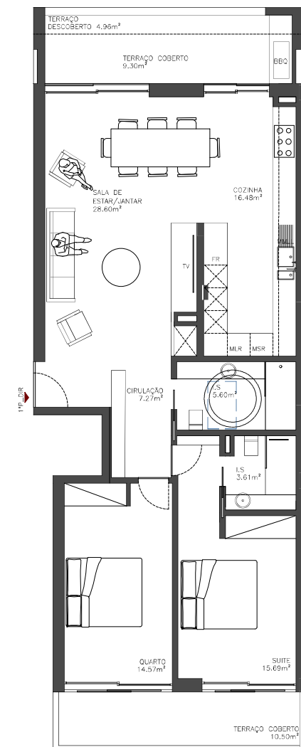
PLANTA LOTE12_ 1º direito_1º piso
