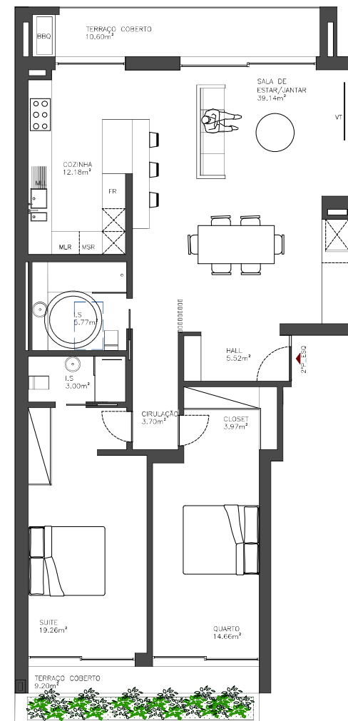
PLANTA LOTE12 _ 2º esquerdo_2º piso
