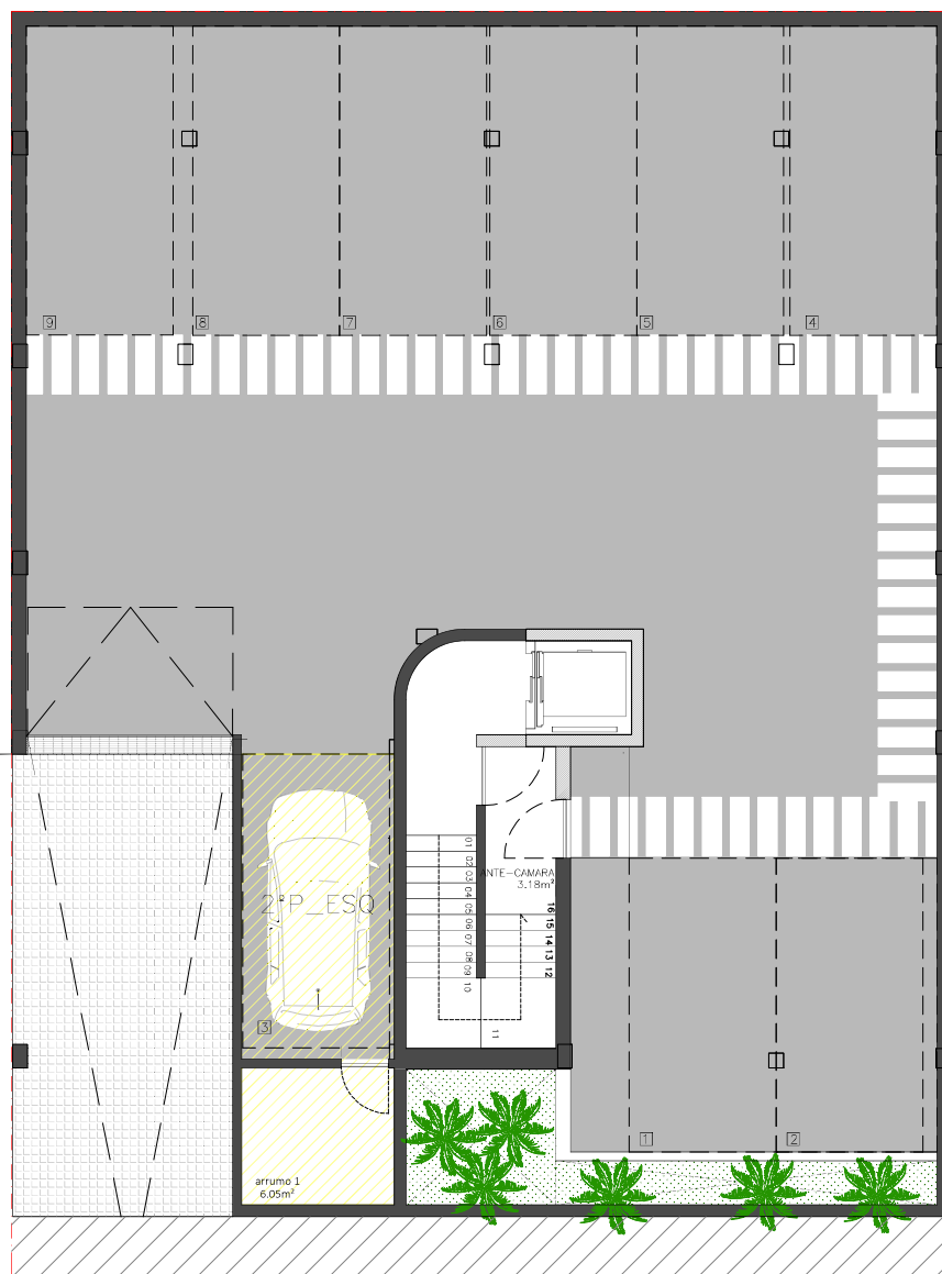
PLANTA DA CAVE LOTE 12_2º esquerdo_2º piso
