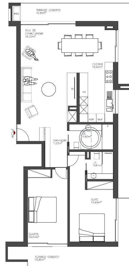
PLANTA LOTE12 _ 3º direito_3º piso
