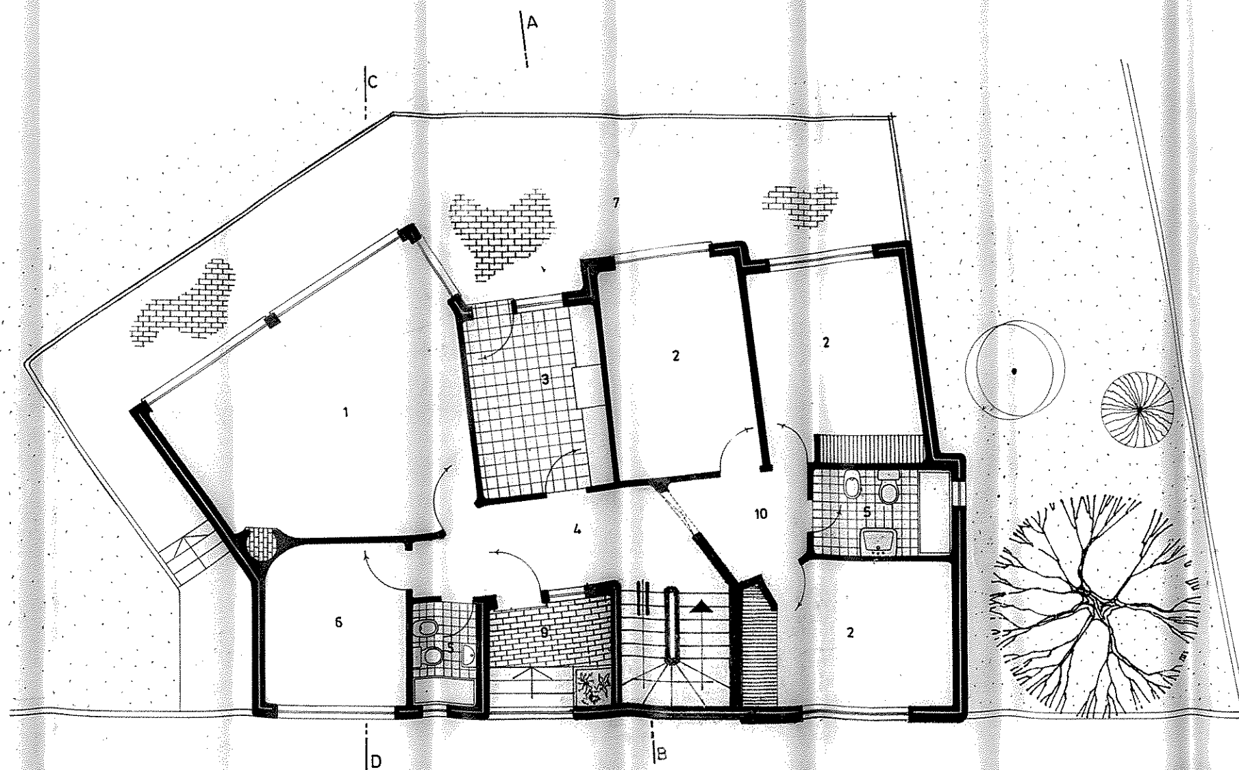
PLANTA DO R. CHÃO
