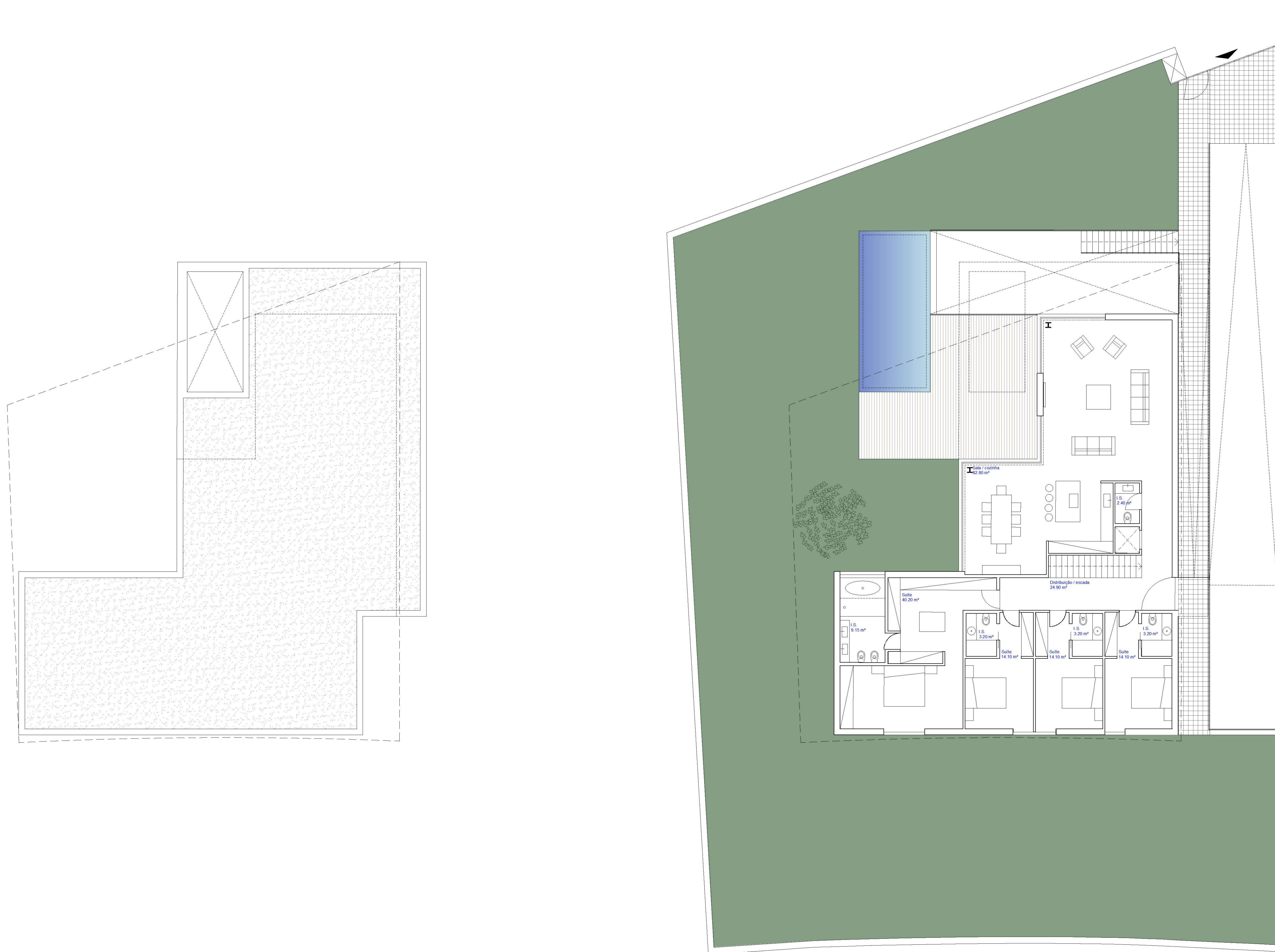
Piso 0 - 247,70 m 2
