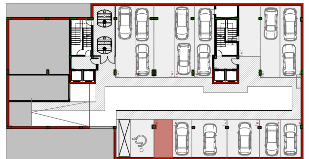
Fracção D - Garagem Planta de Localização
