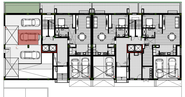
Fracção I - Garagem Planta de Localização
