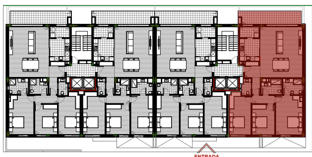
Fracção G - Habitação Planta de Localização
