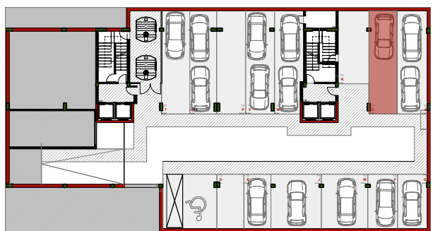
Fracção O - Garagem Planta de Localização
