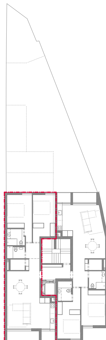
piso 1
