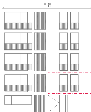
alçado principal
