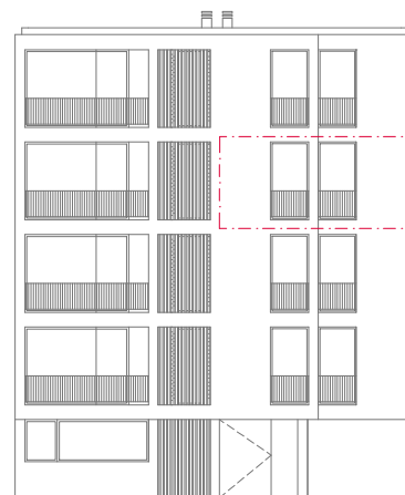
alçado principal
