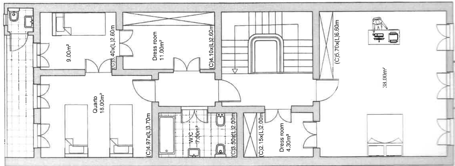
Planta do 3.º Andar
