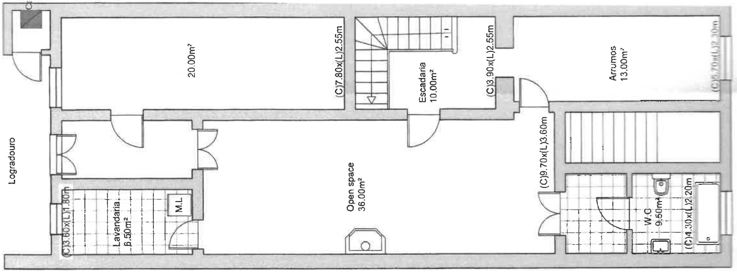
Planta do 1.º Andar
