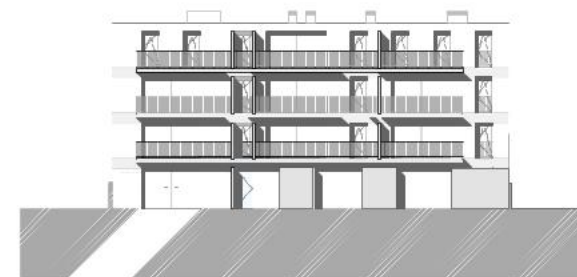
ALÇADO TARDOZ
