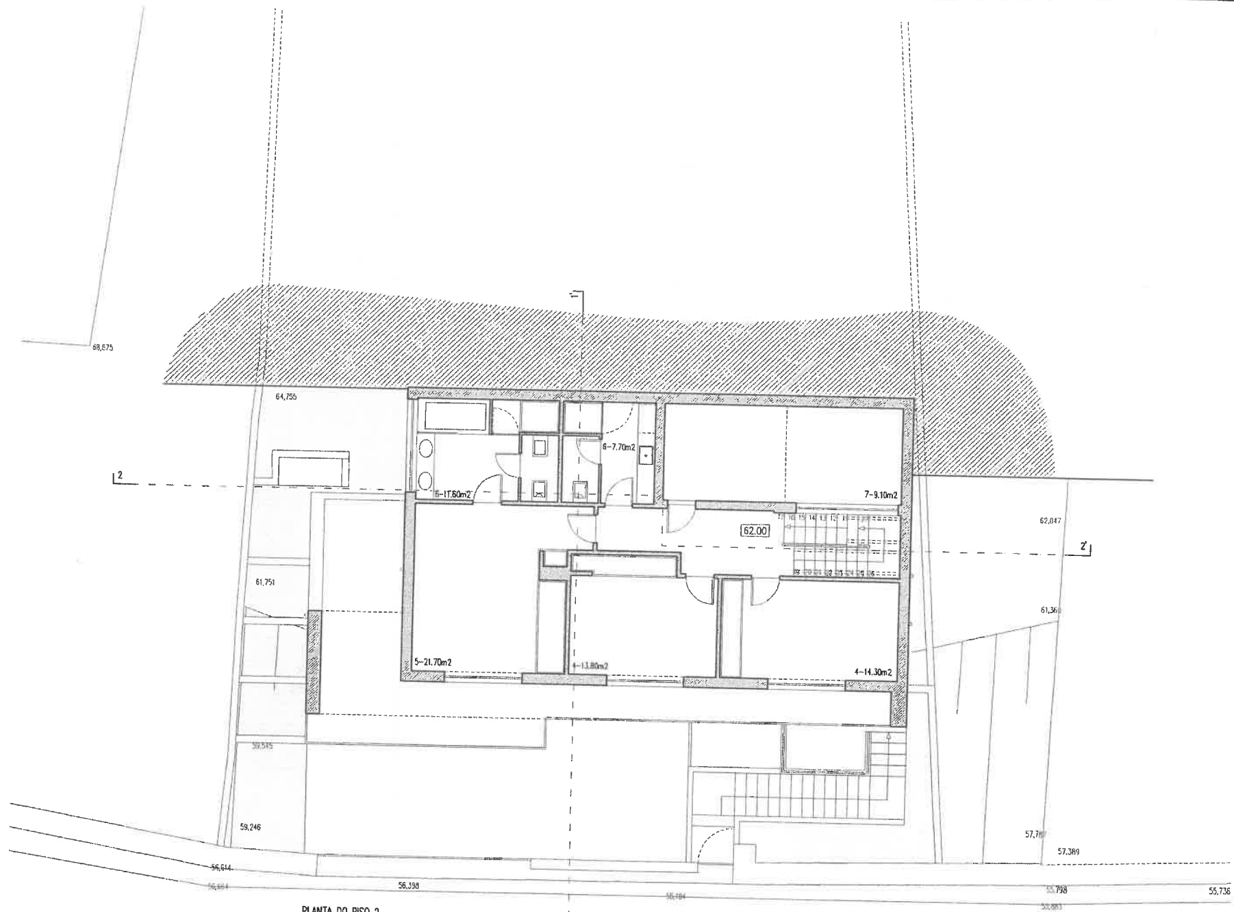
PLANTA DO PISO 2
