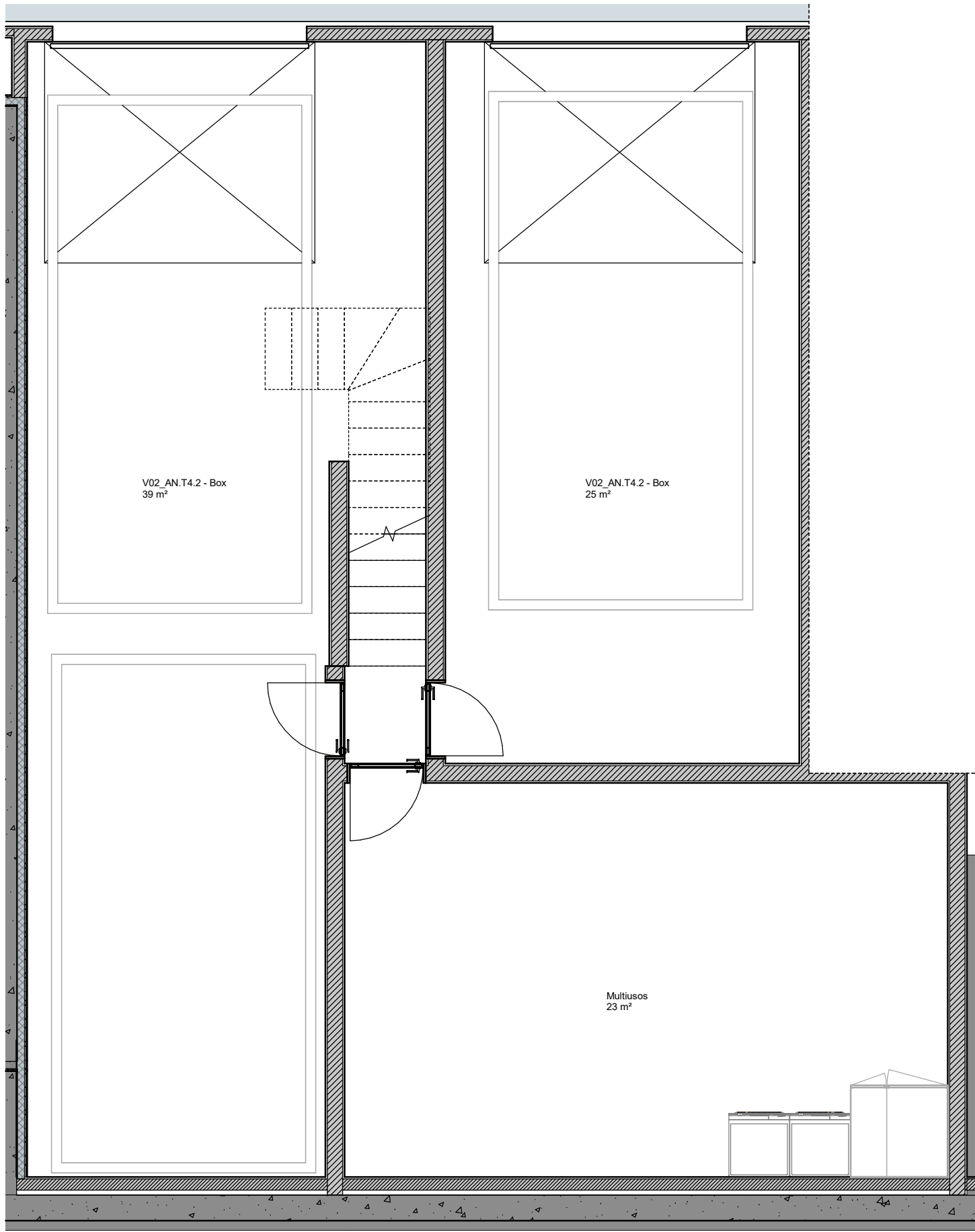
V02_AN.T4.2 - Box 1 : 50
