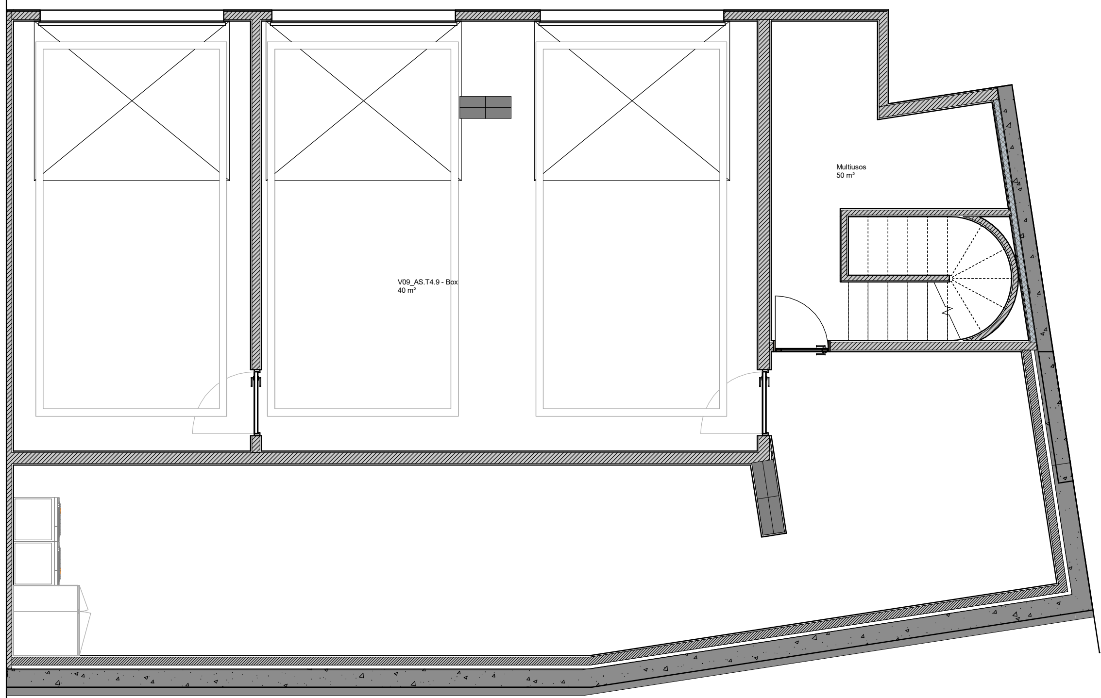
V09_AS.T4.9 - Box 1:50
