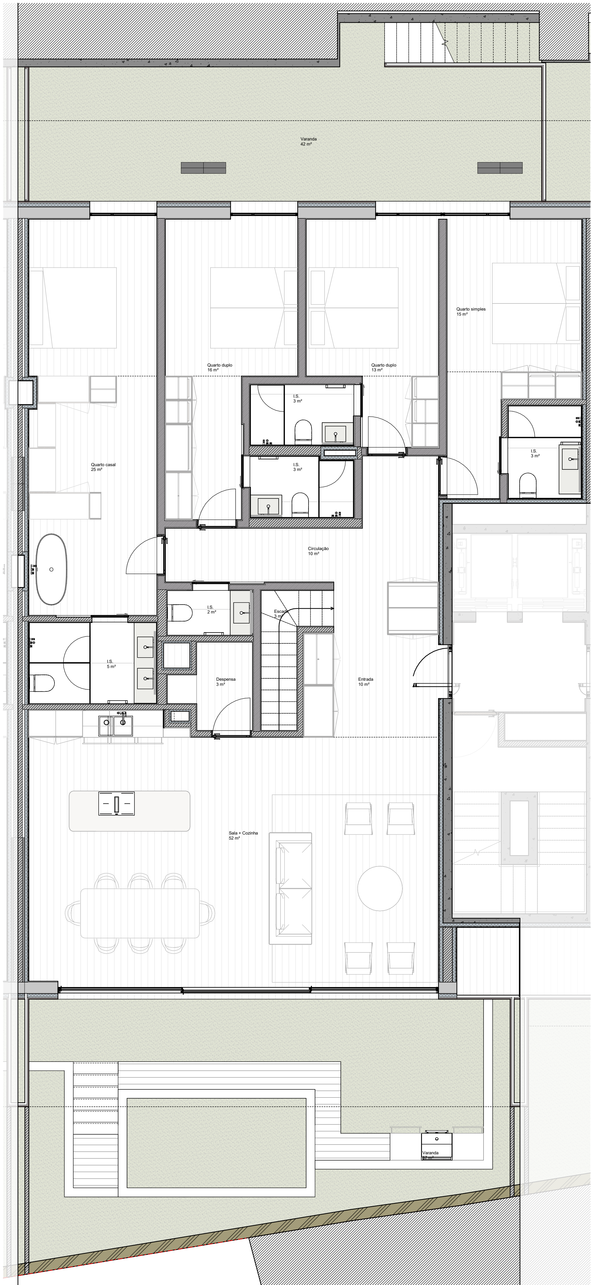
V07_AS.T4.7 1:50
