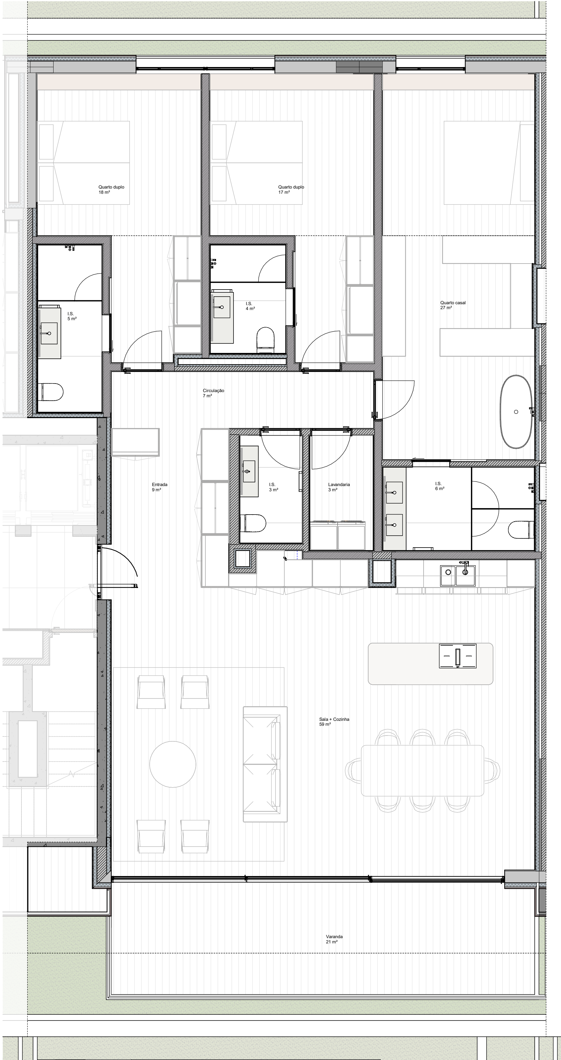
108_AS.T3.4 1 : 50
