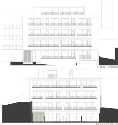
Alçado Posterior
