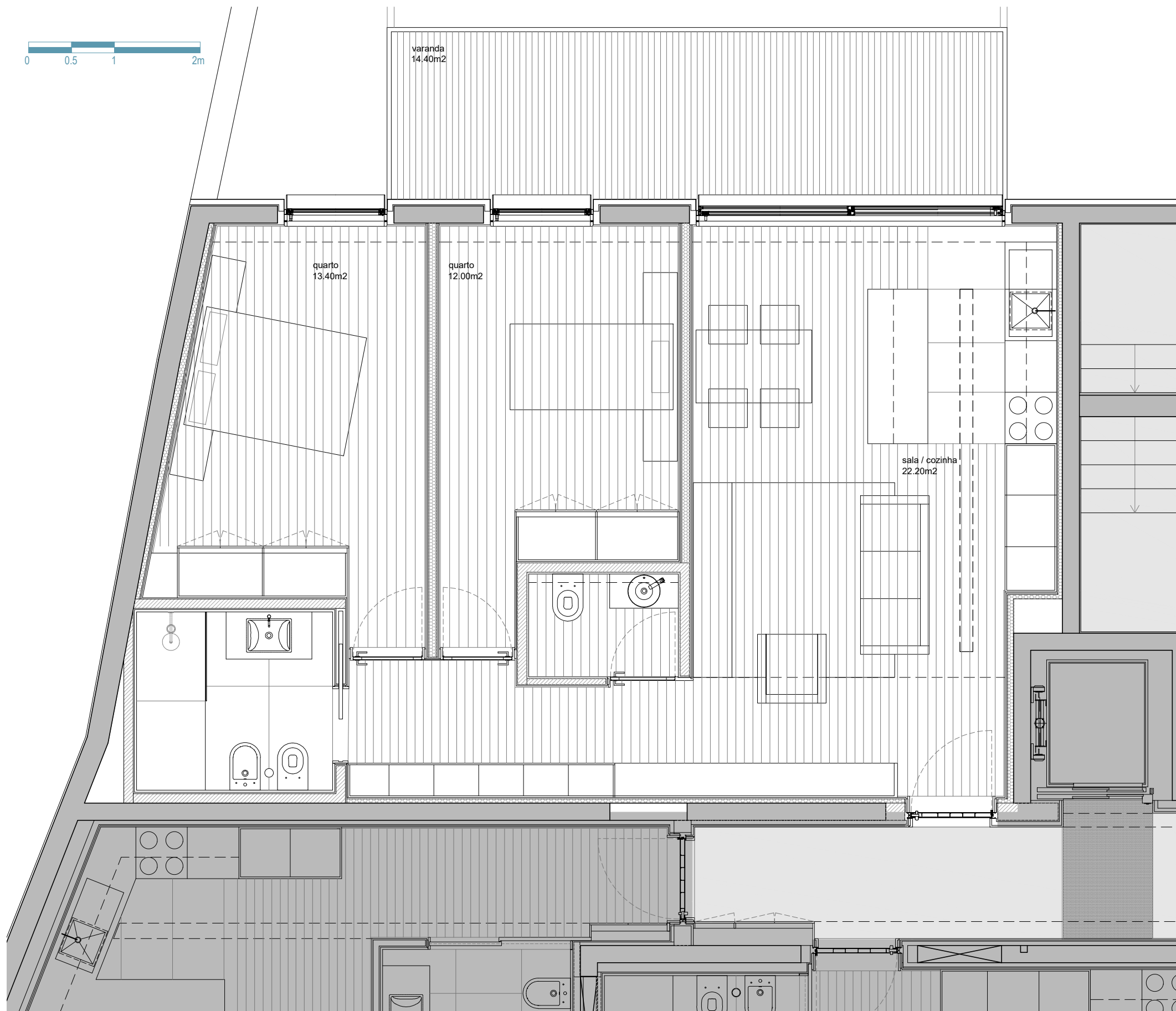
Planta do Piso 2
