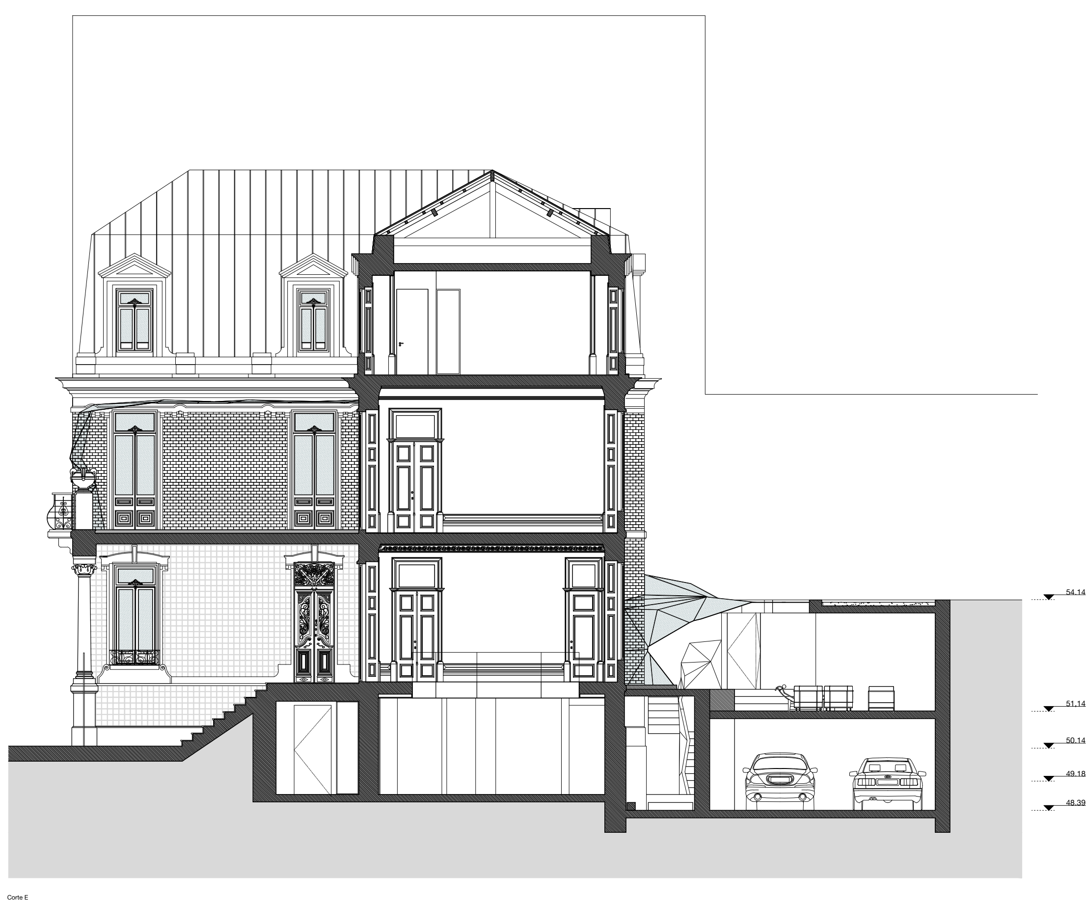
Corte E
