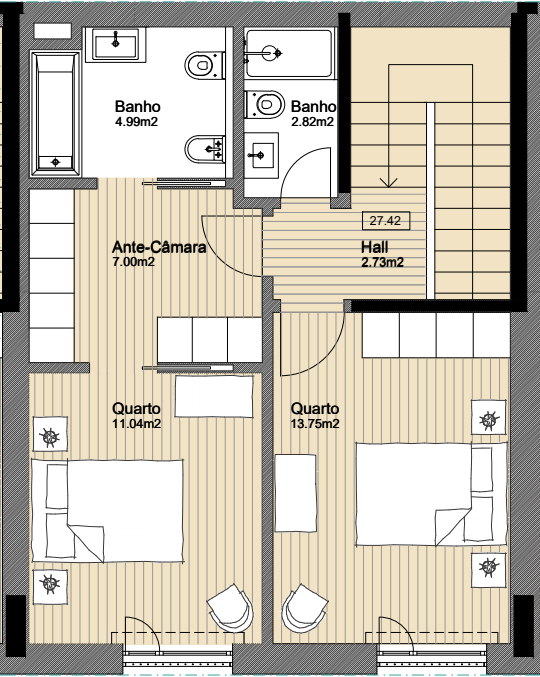
PLANTA DO PISO 1
