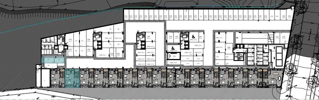
PISO 0 | ÉTAGE 0 | FLOOR 0
