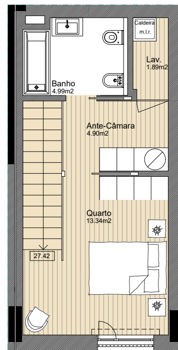
PLANTA DO PISO 1
