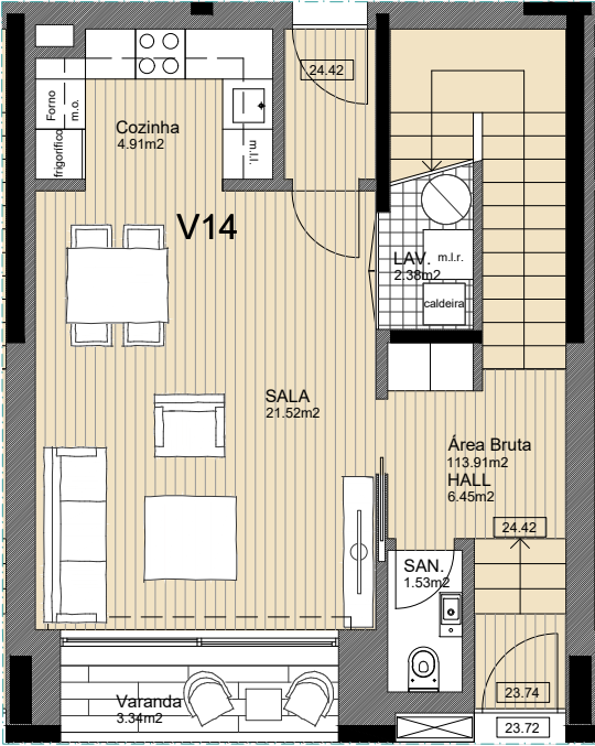
PLANTA DA CAVE 0
