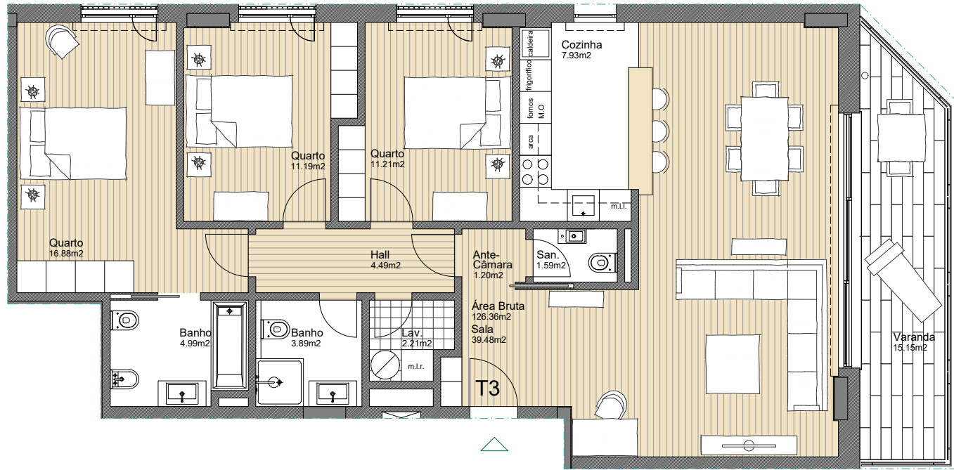
PLANTA DO 4º PISO
