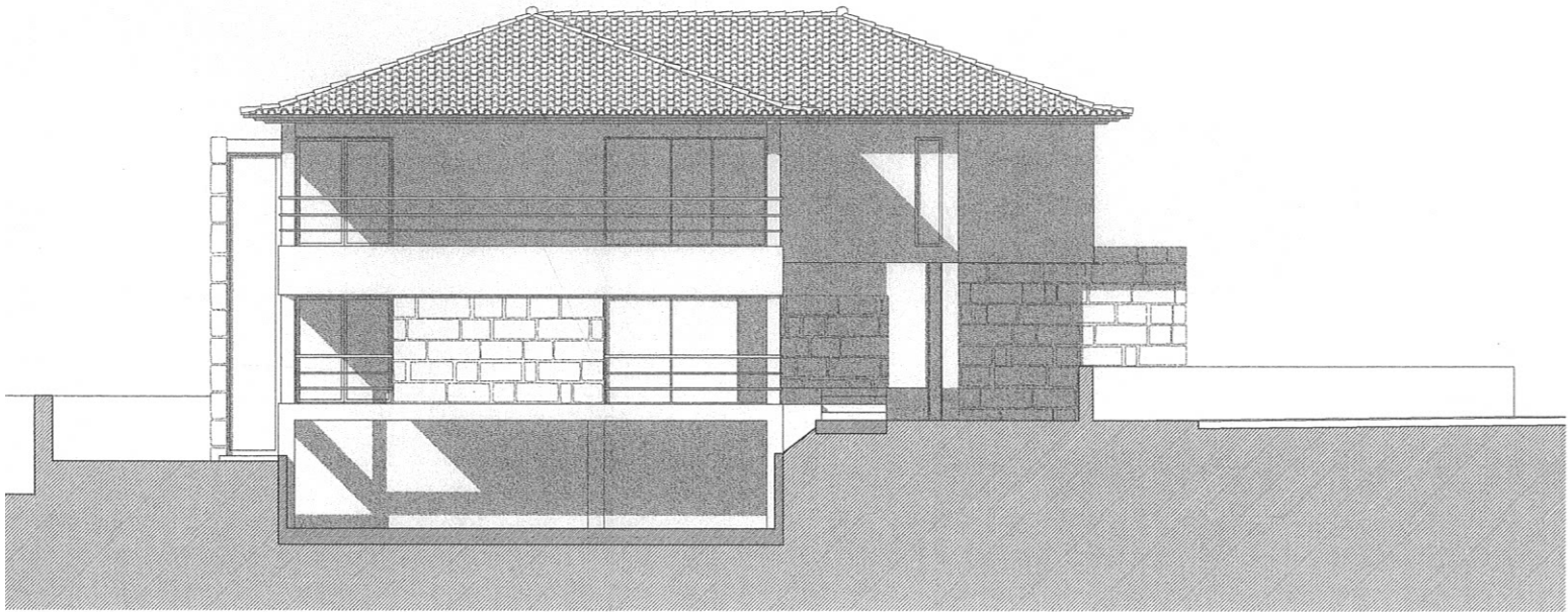
ALÇADO POENTE
