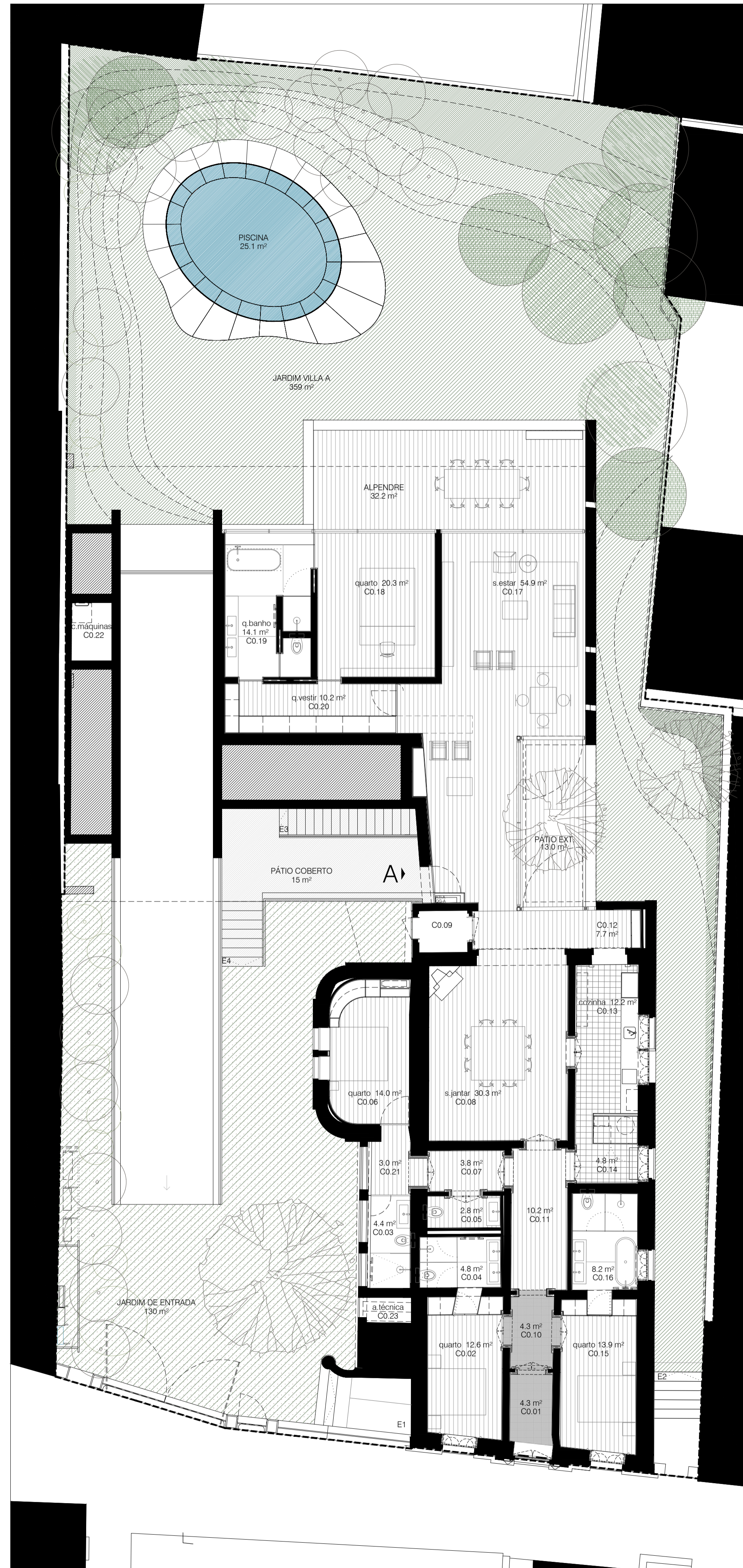
Planta do Piso 0
