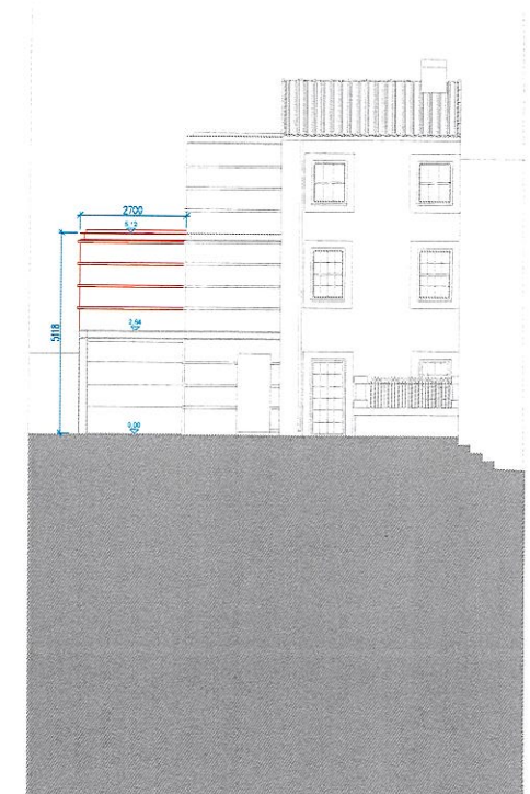
ALÇADO NORTE (PRINCIPAL) | PROPOSTA
