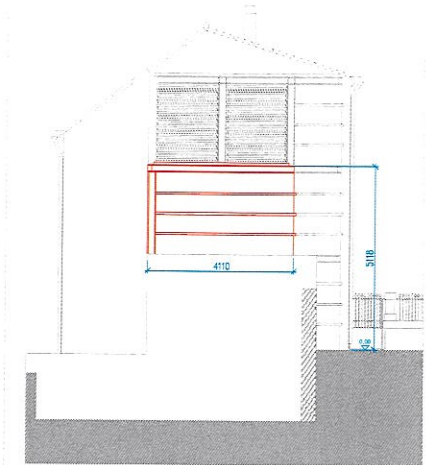
ALÇADO NASCENTE | PROPOSTA
