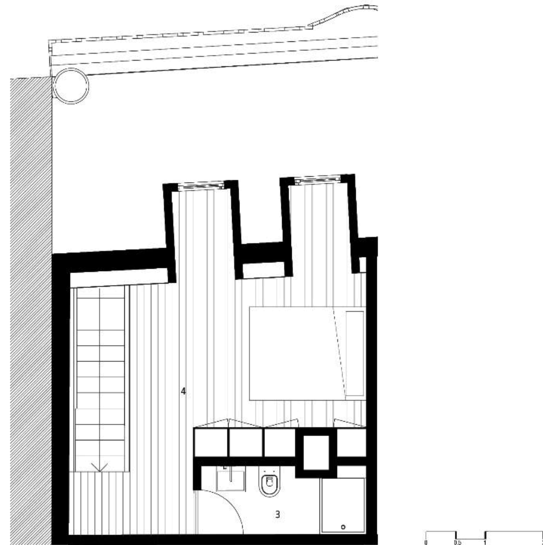
Planta Piso 2
