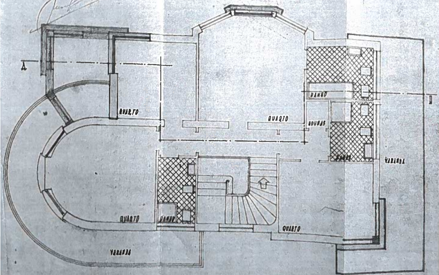
PLANTA DO ANDAR
