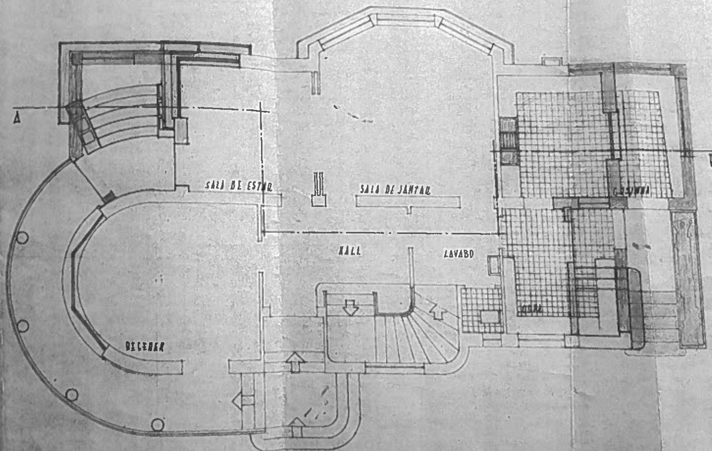
PLANTA DO R. 1.º ANDAR
