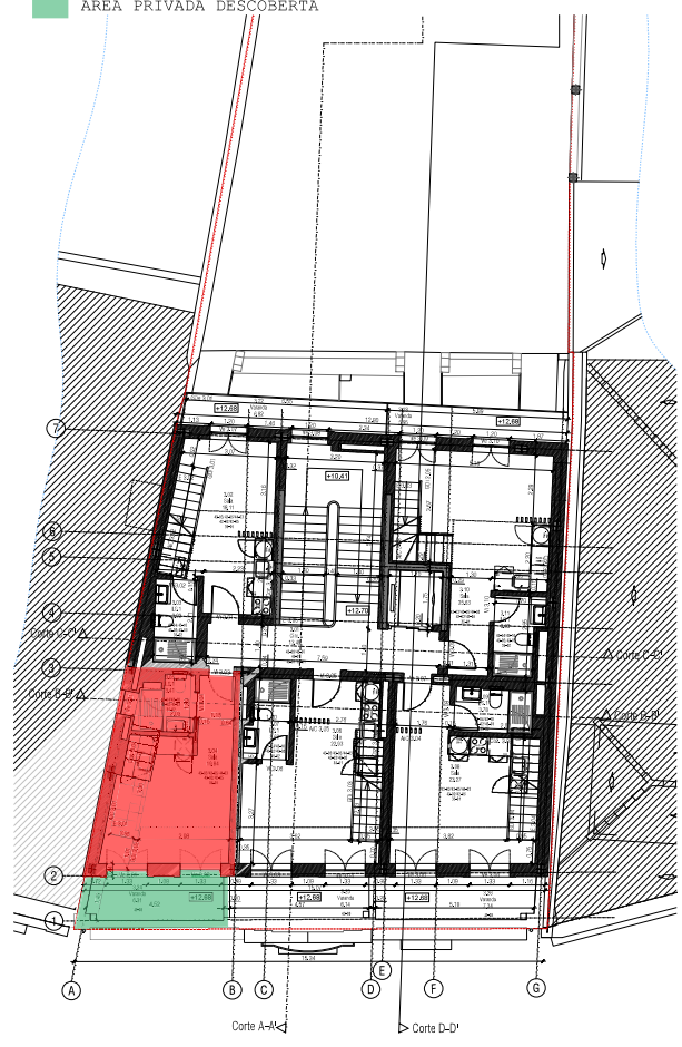
PLANTA DO 3º ANDAR (cota 12,70 m) BLOCO A
