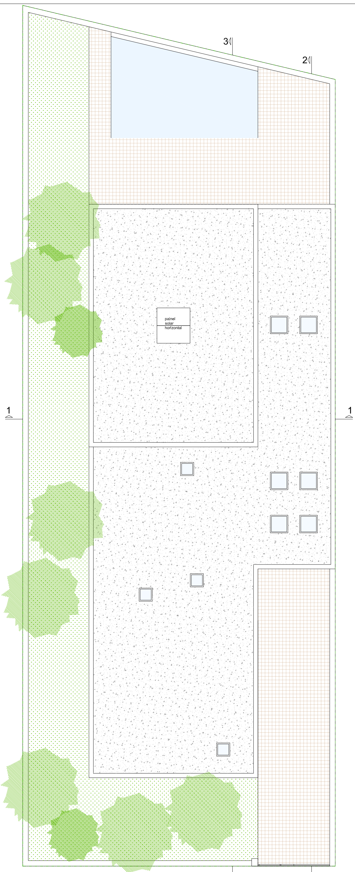
2/1 PLANTA - COBERTURA
