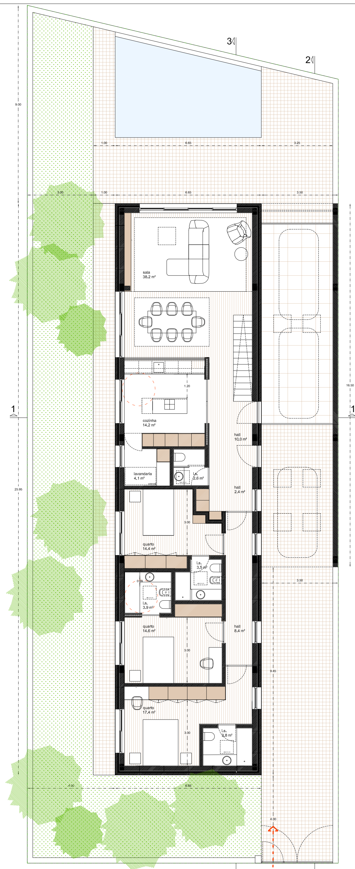
2/1 PLANTA - PISO 0
