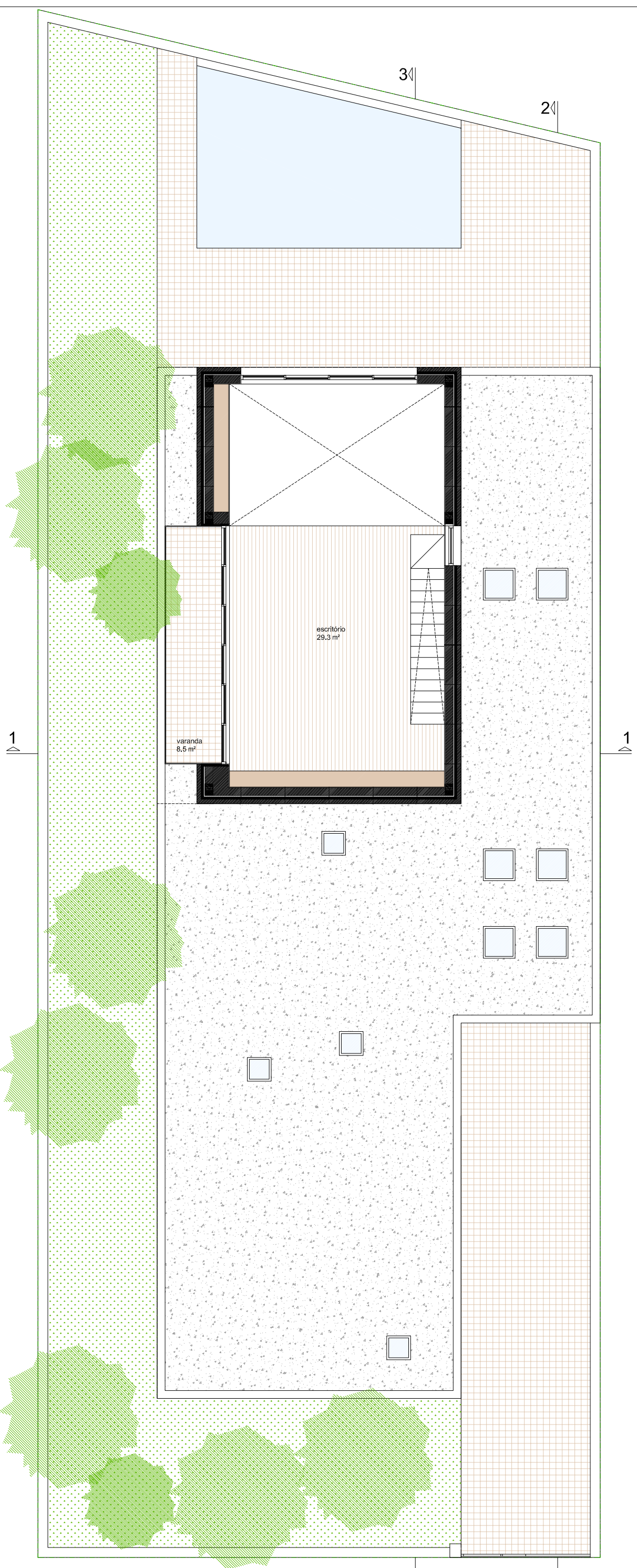
2/1 PLANTA - PISO 1
