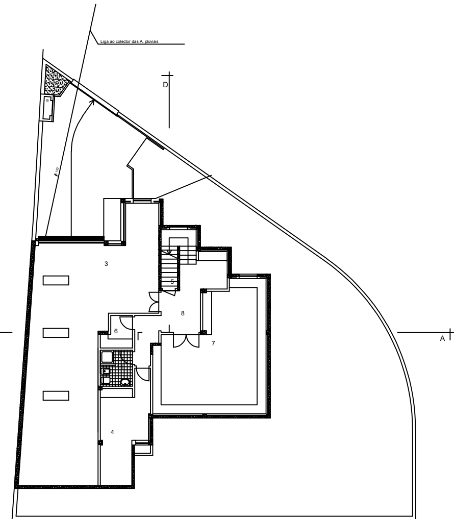
PLANTA DA CAVE
