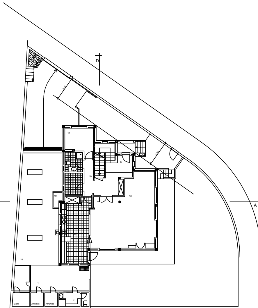
PLANTA DO R/CHAO
