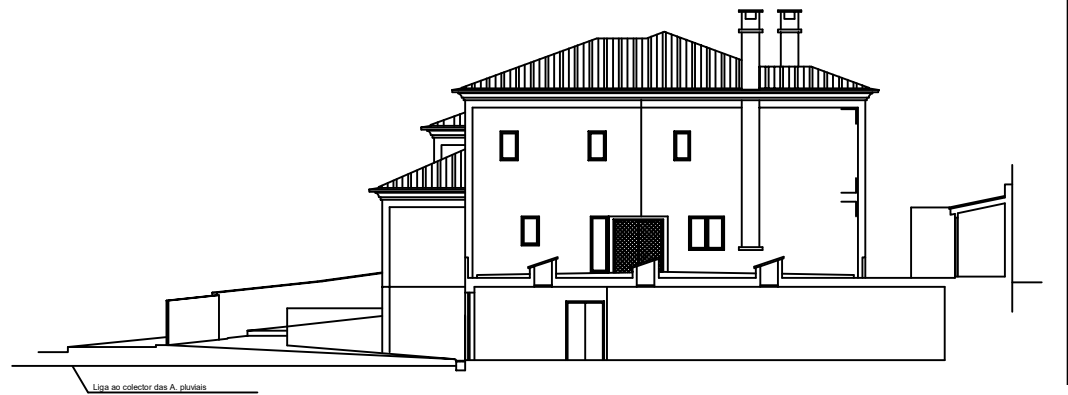
ALCADO NORTE
