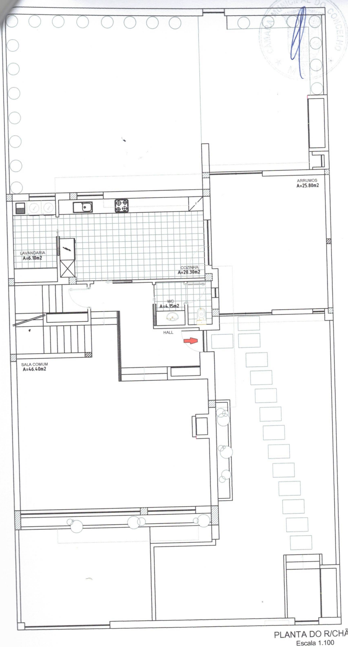
3b - PLANTA SIMPLIFICADA DO PISO DE ACESSO AO FOGO
