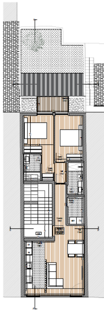
PLANTA PISO 2
