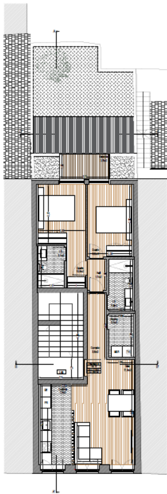
PLANTA PISO 1
