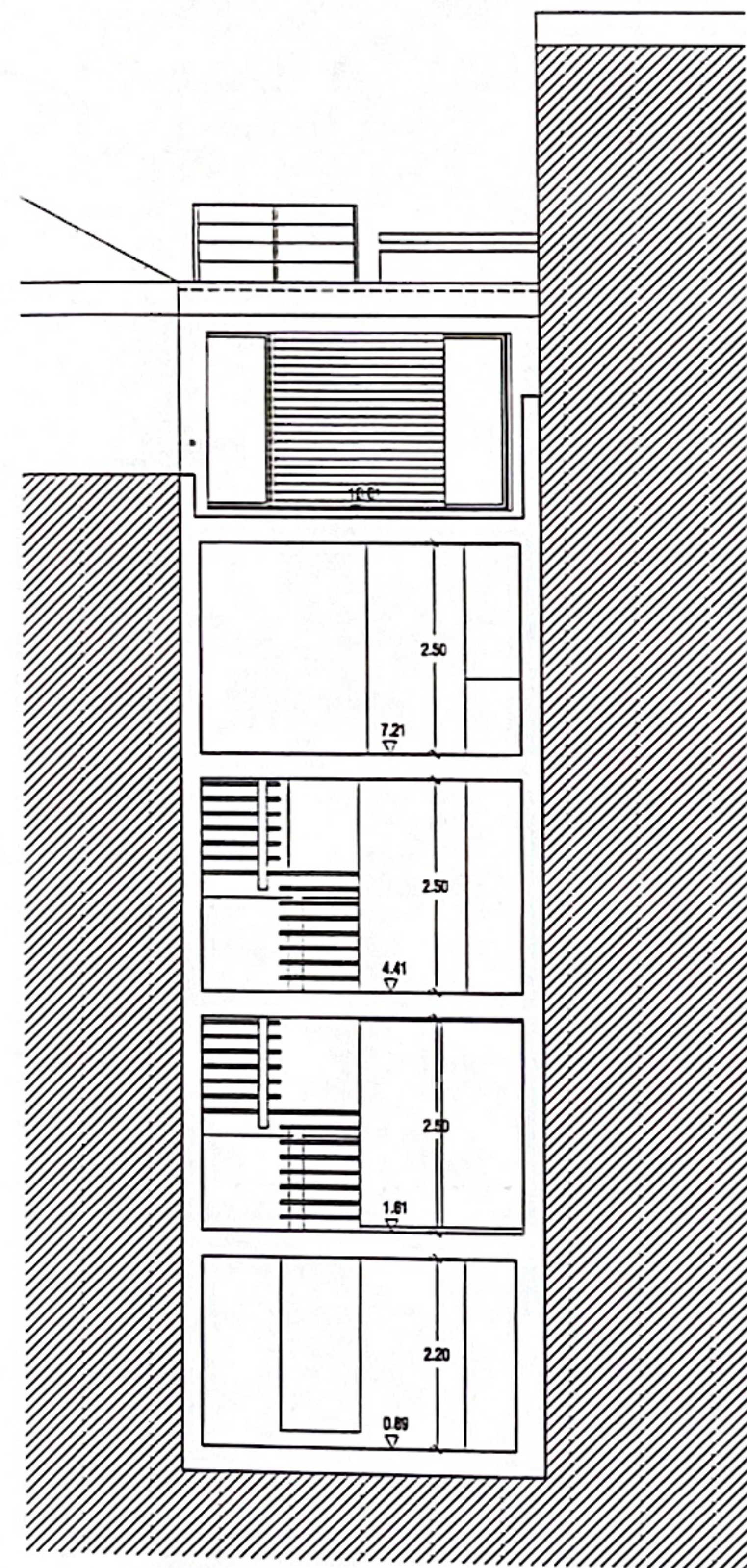
CORTE 2
