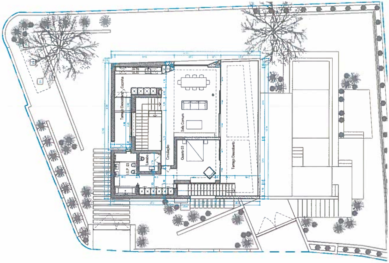
PLANTA DO PISO 1
