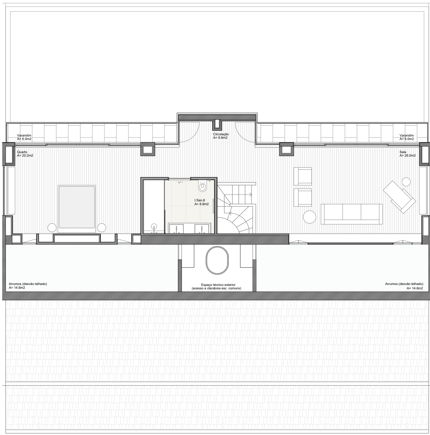
Planta de Piso 05 - Triplex - recuado, esc.1/100
