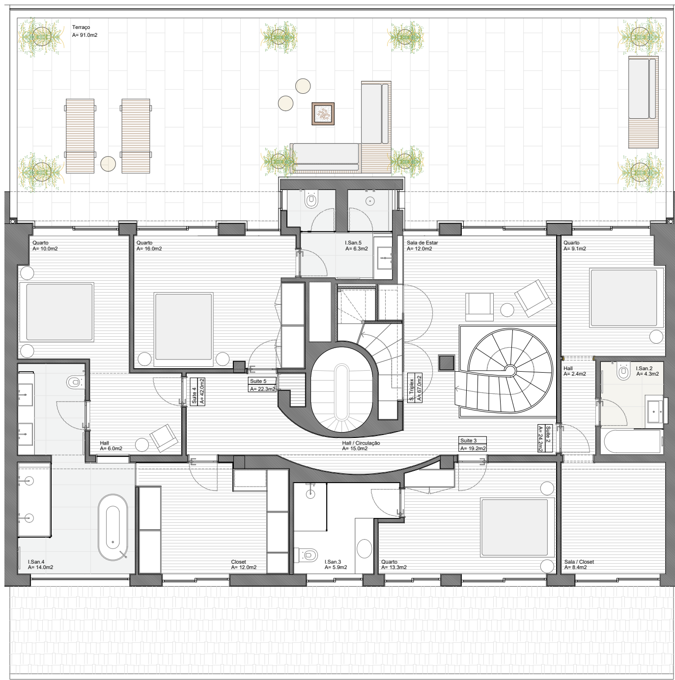
Planta de Piso 04 - recuado, esc. 1/100
