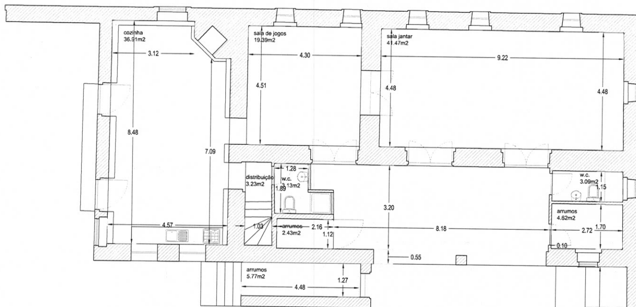
PLANTA DO RÉS DO CHÃO HABITAÇÃO = 200.00 m²
