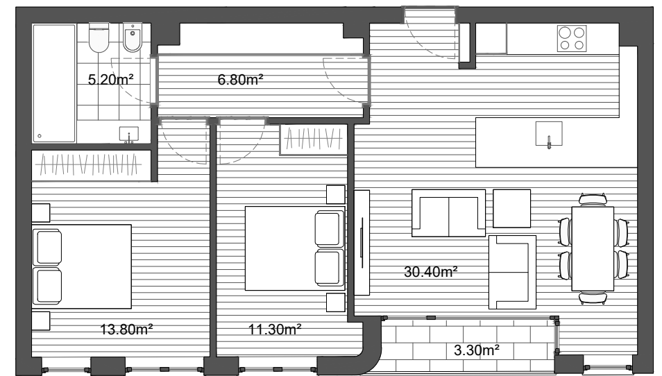
H.1.7 Piso 1
