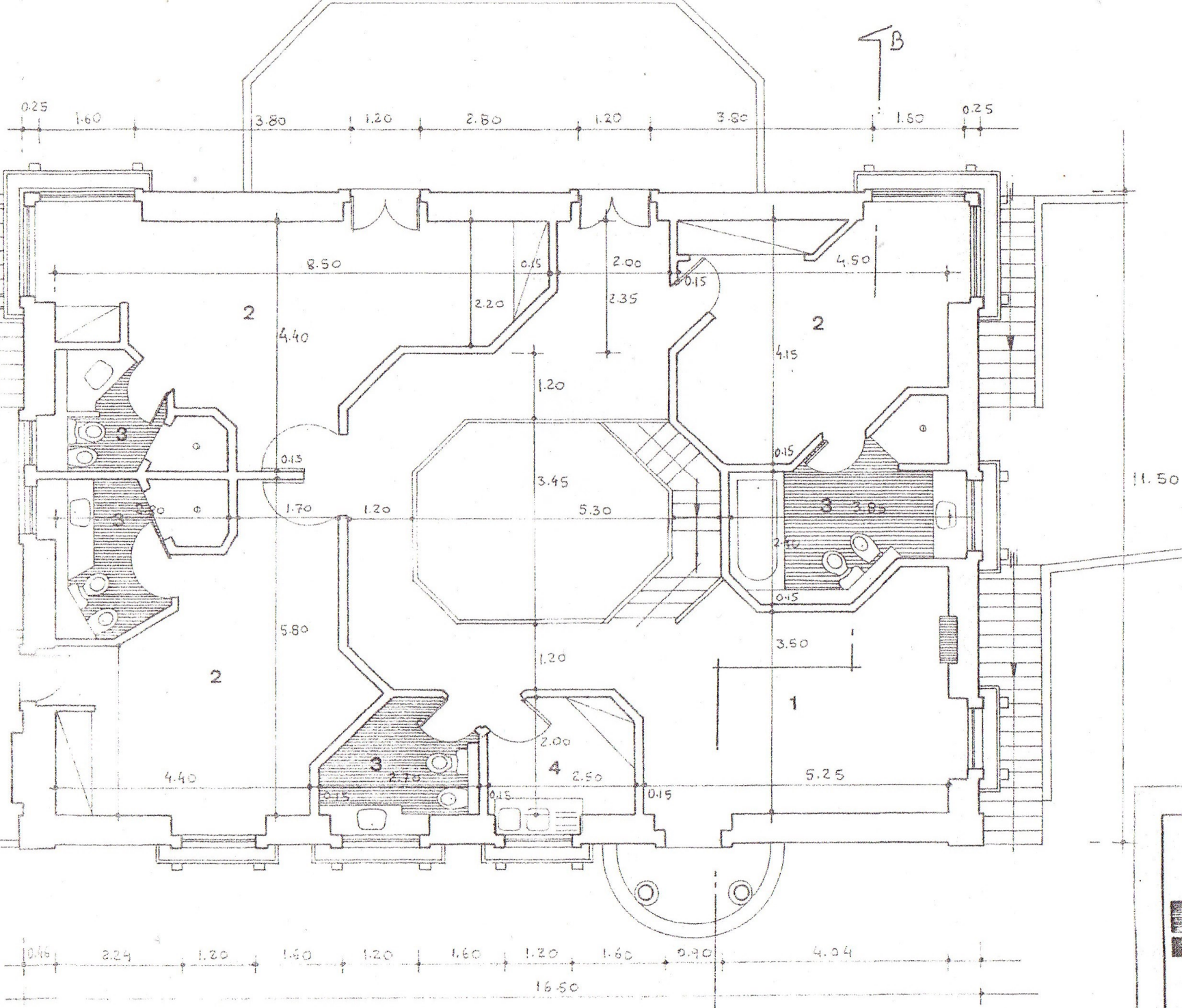
PLANTA DO 3º PISO
