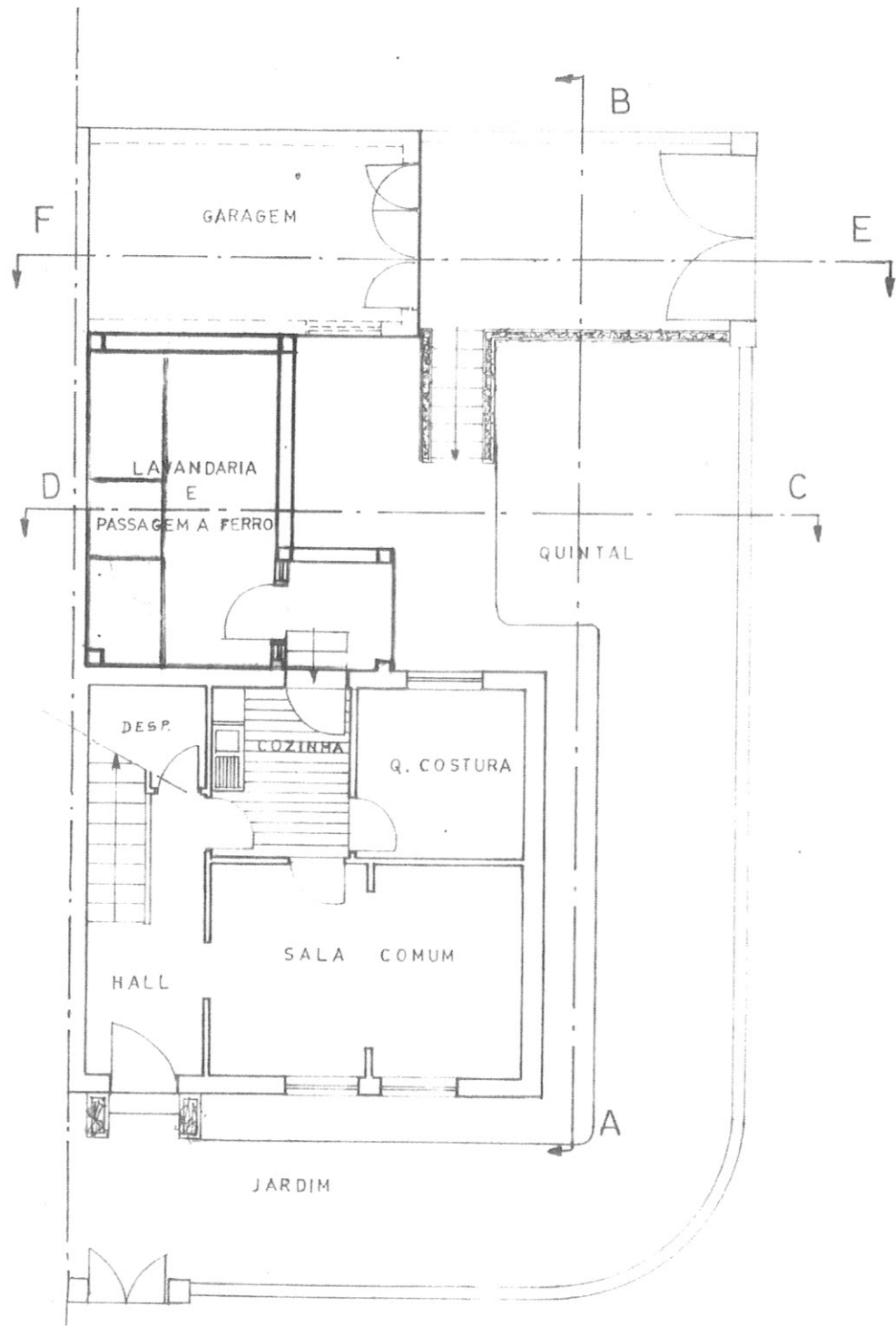
PLANTA DO R.CHÃO
