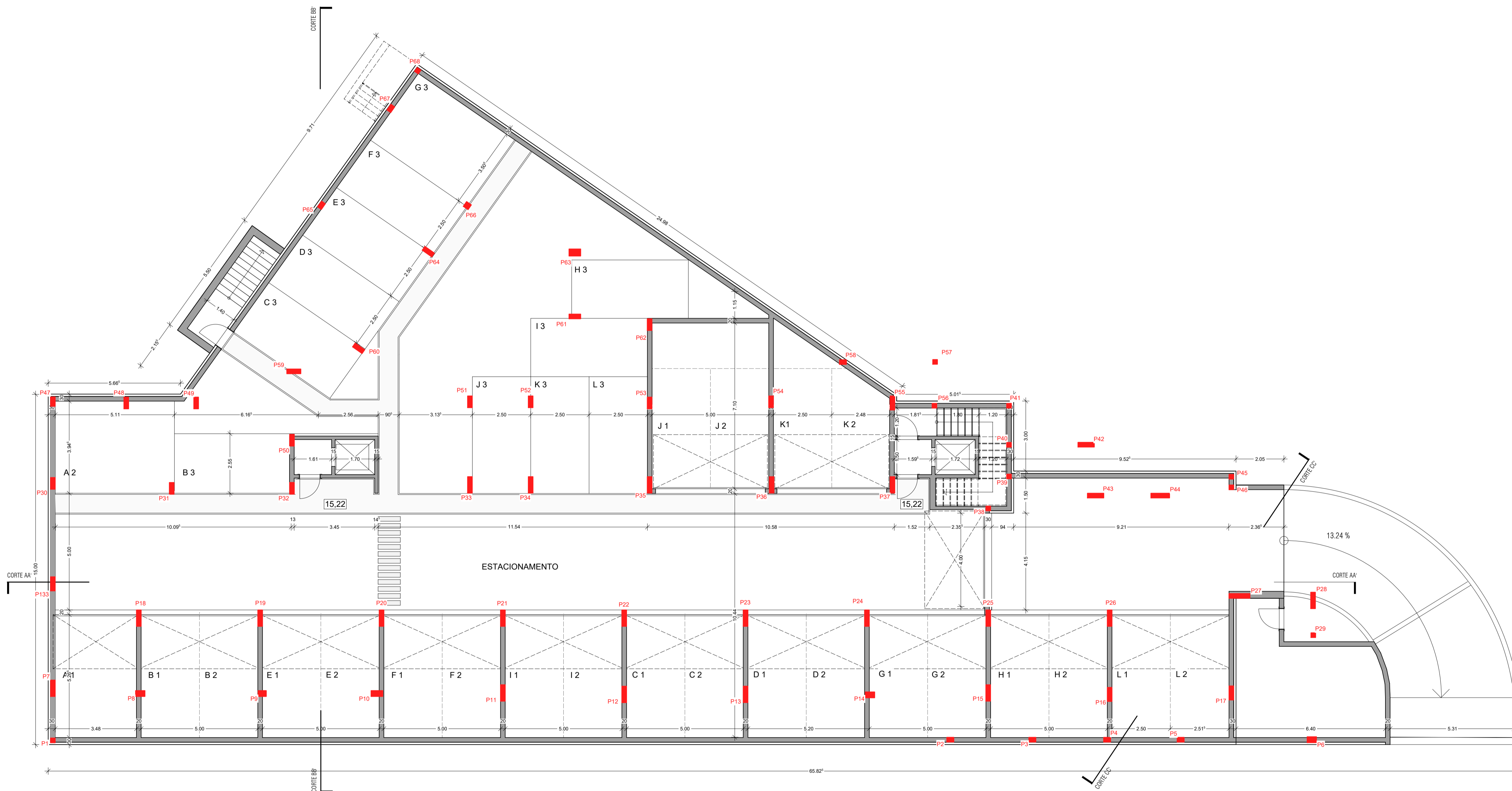
PLANTA PISO CAVE
