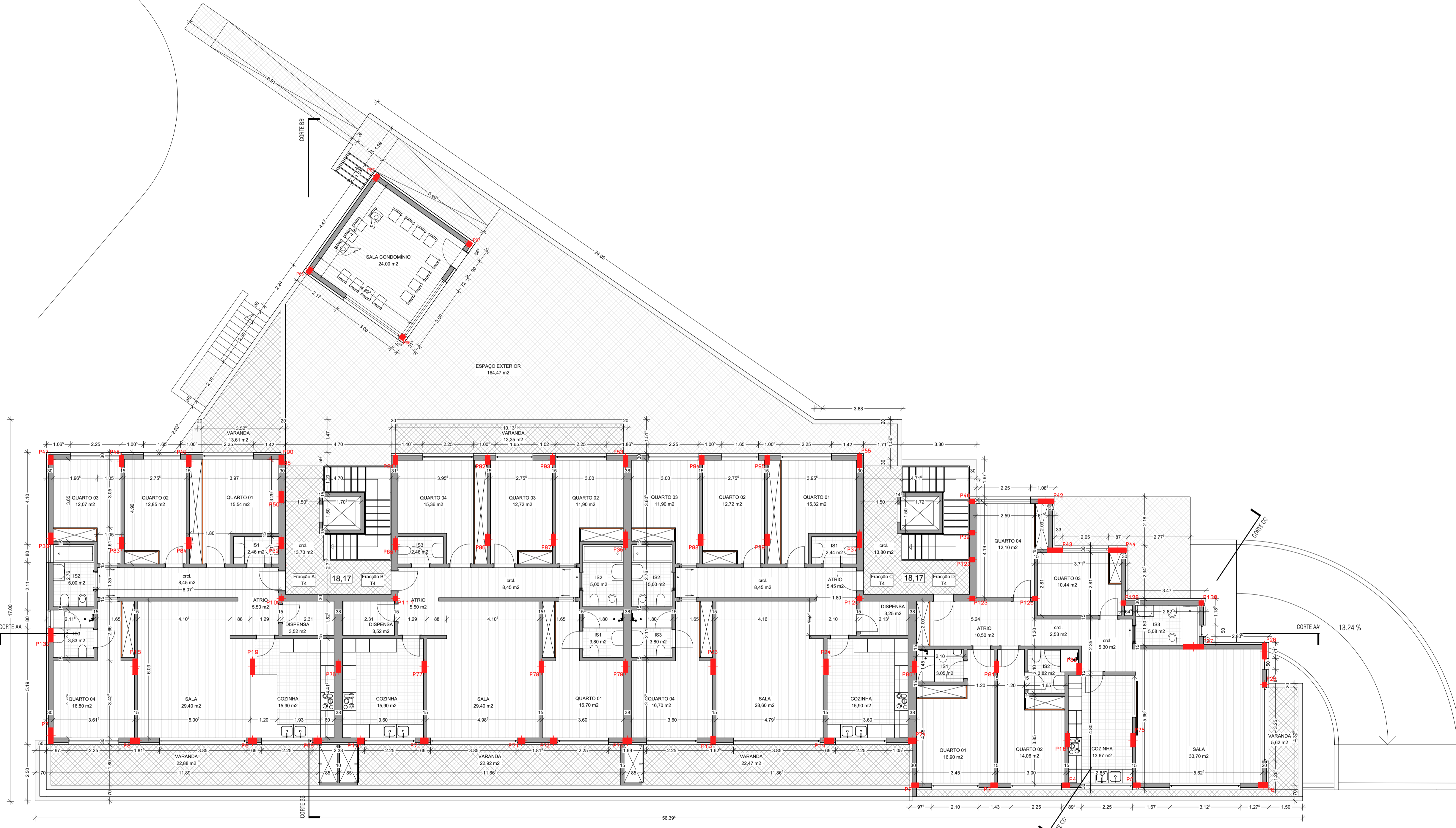
PLANTA PISO 00
