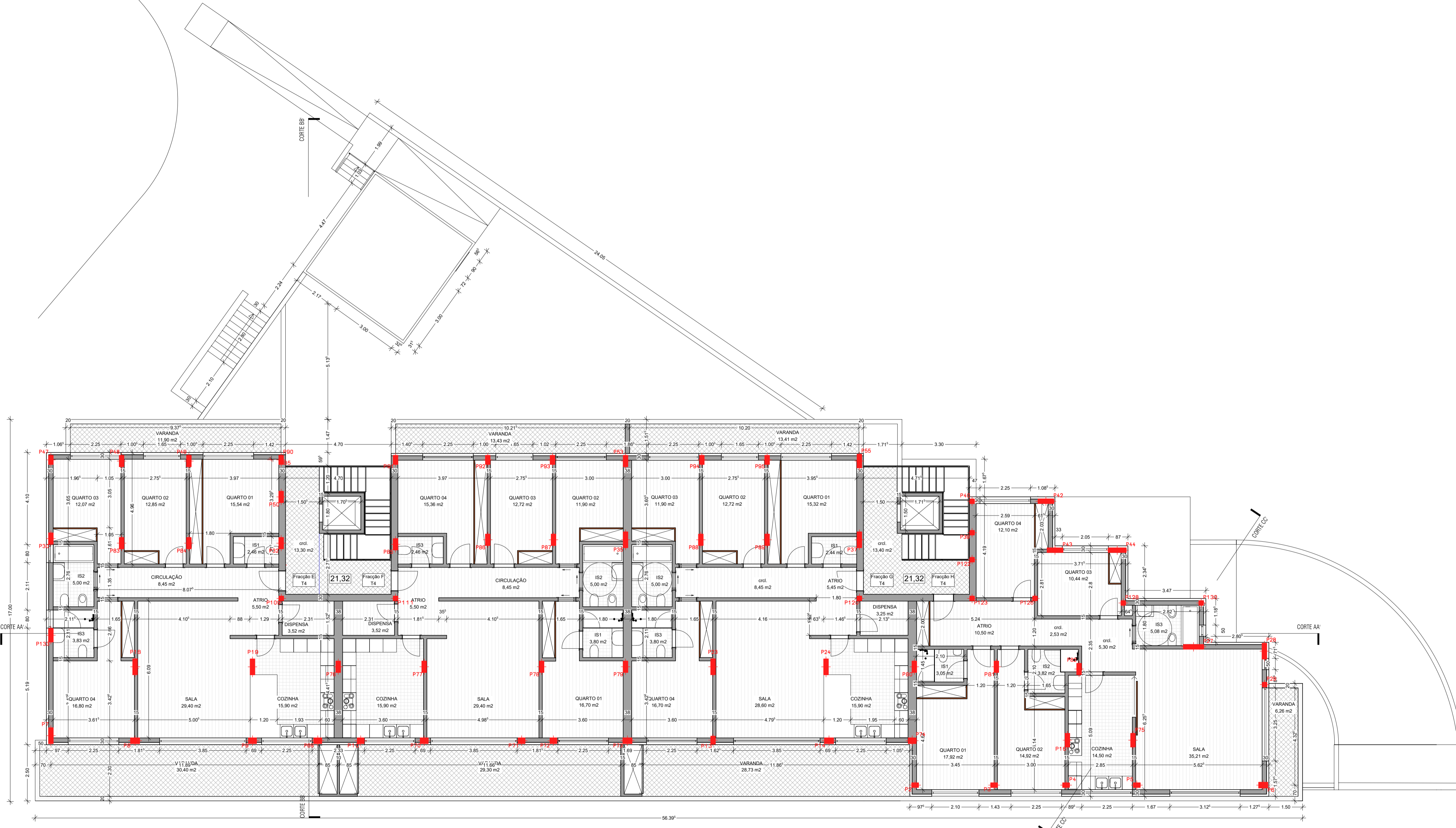
PLANTA PISO 01
