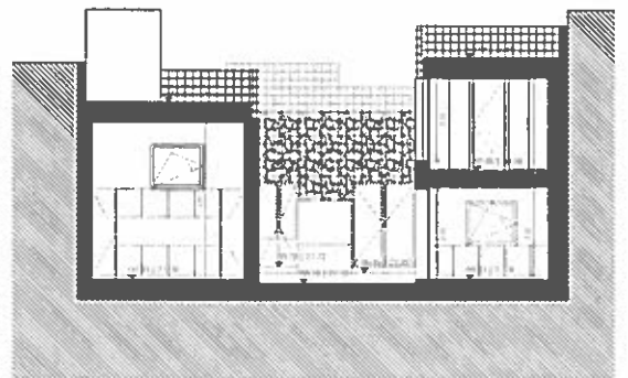
CORTE C3
